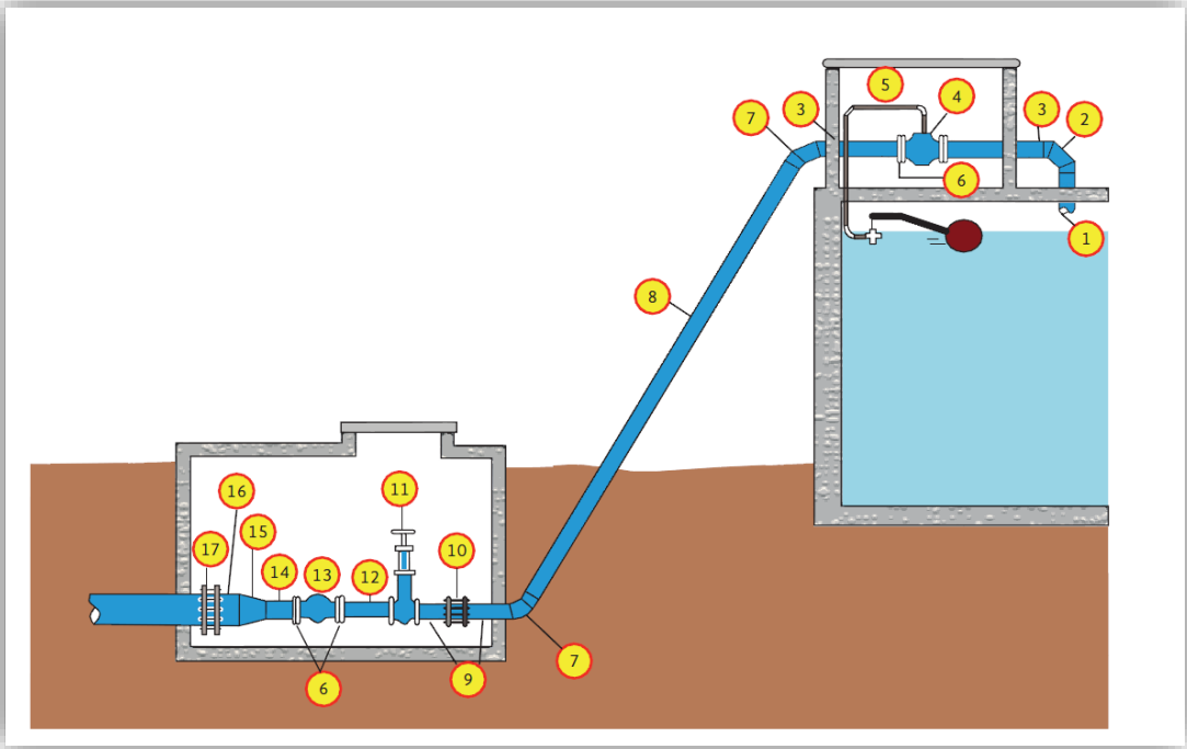
Esquema: Tanque superficial, Fontanería de llegada.
