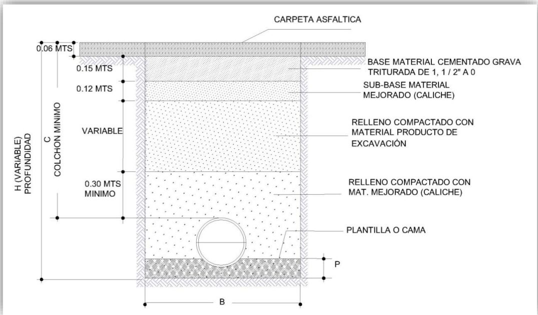
Esquema. Relleno de Zanja en Vialidad de Concreto.
