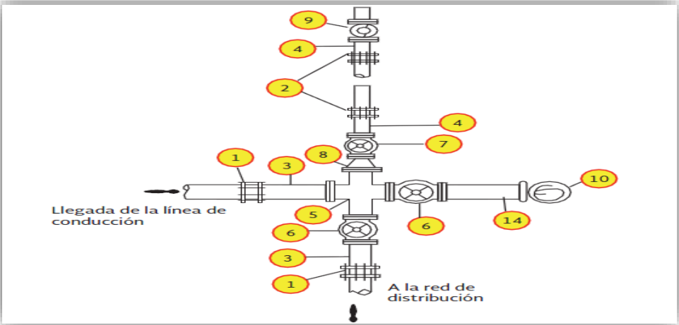
Esquema: Tanque Elevado. Arreglo de fontanería entrada-salida (elevación).
